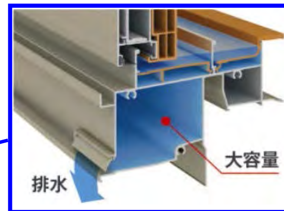
下部断面
