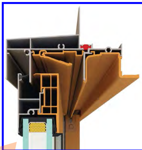
上部断面
